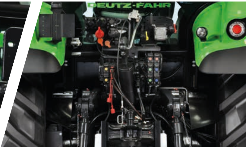
> Bis zu 5 elektrische Steuergeräte am Heck.
